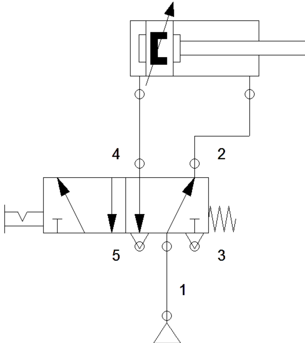
Esquema 02: Accionamiento directo sistema neumático actuador doble efecto
